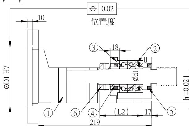
剖面圖 AF-AF
