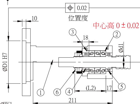
剖面圖 AF-AF
