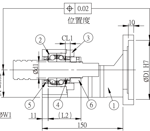
剖面圖 V-V
