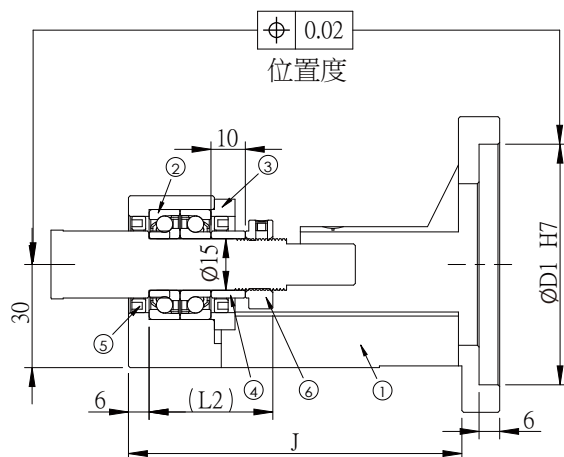
剖面圖 V-V
