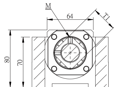
剖面圖 U-U
