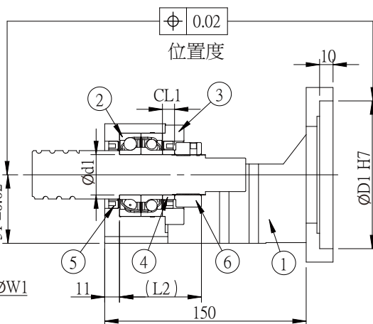
剖面圖 V-V
